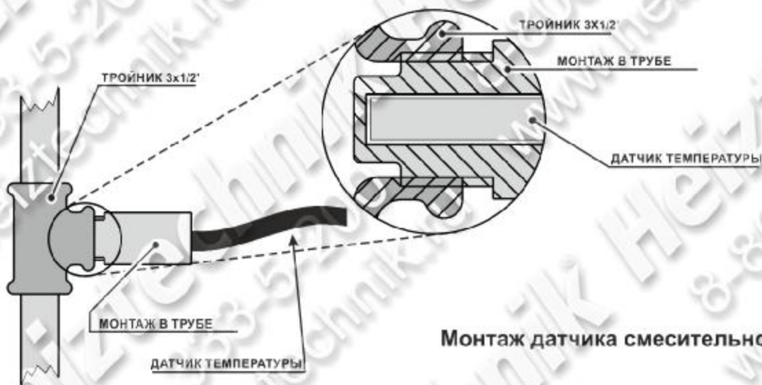
Монтаж уличного датчика
