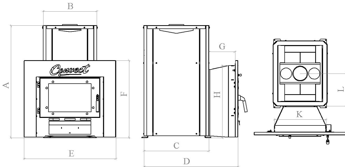
Рис. 1 Основные размеры печи CONVECT
