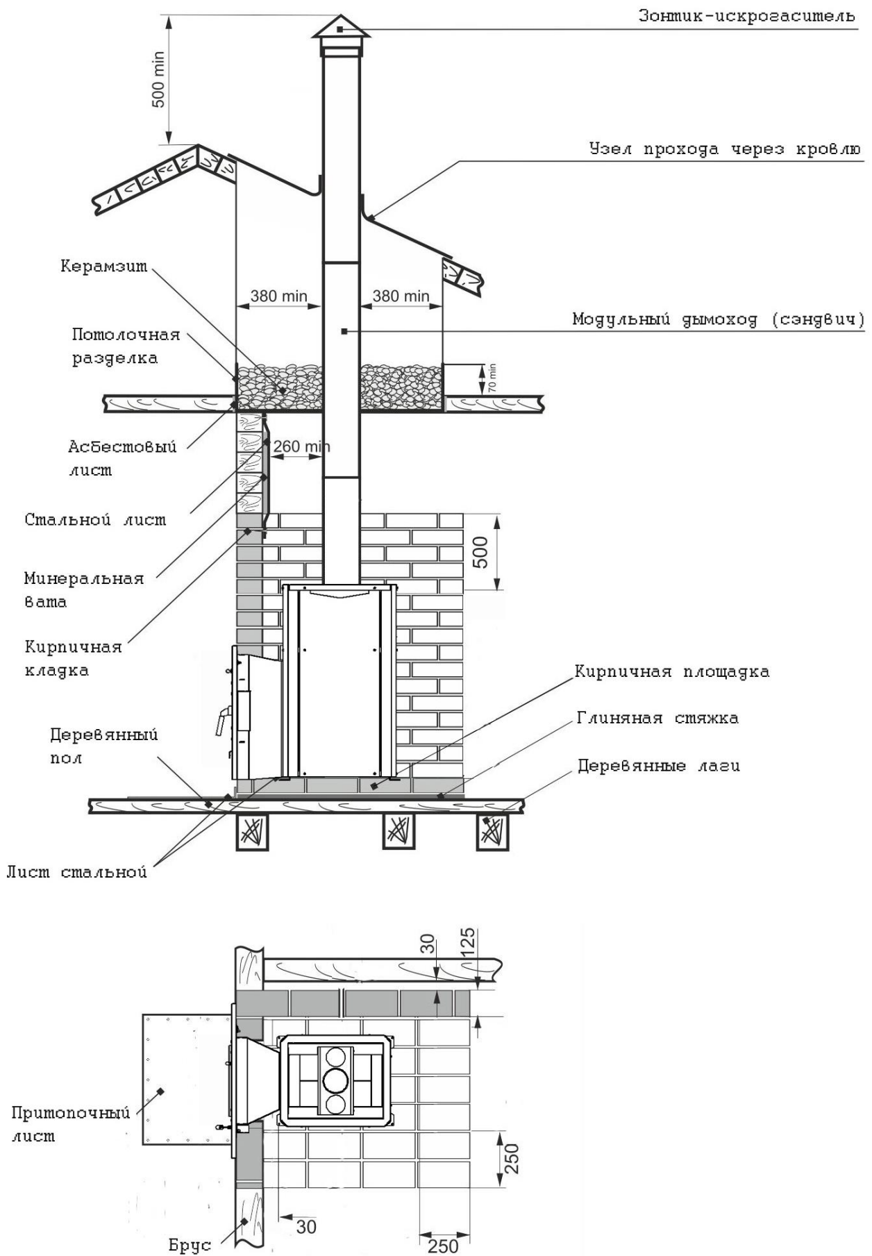
Рис. 3 Монтаж печи CONVECT
