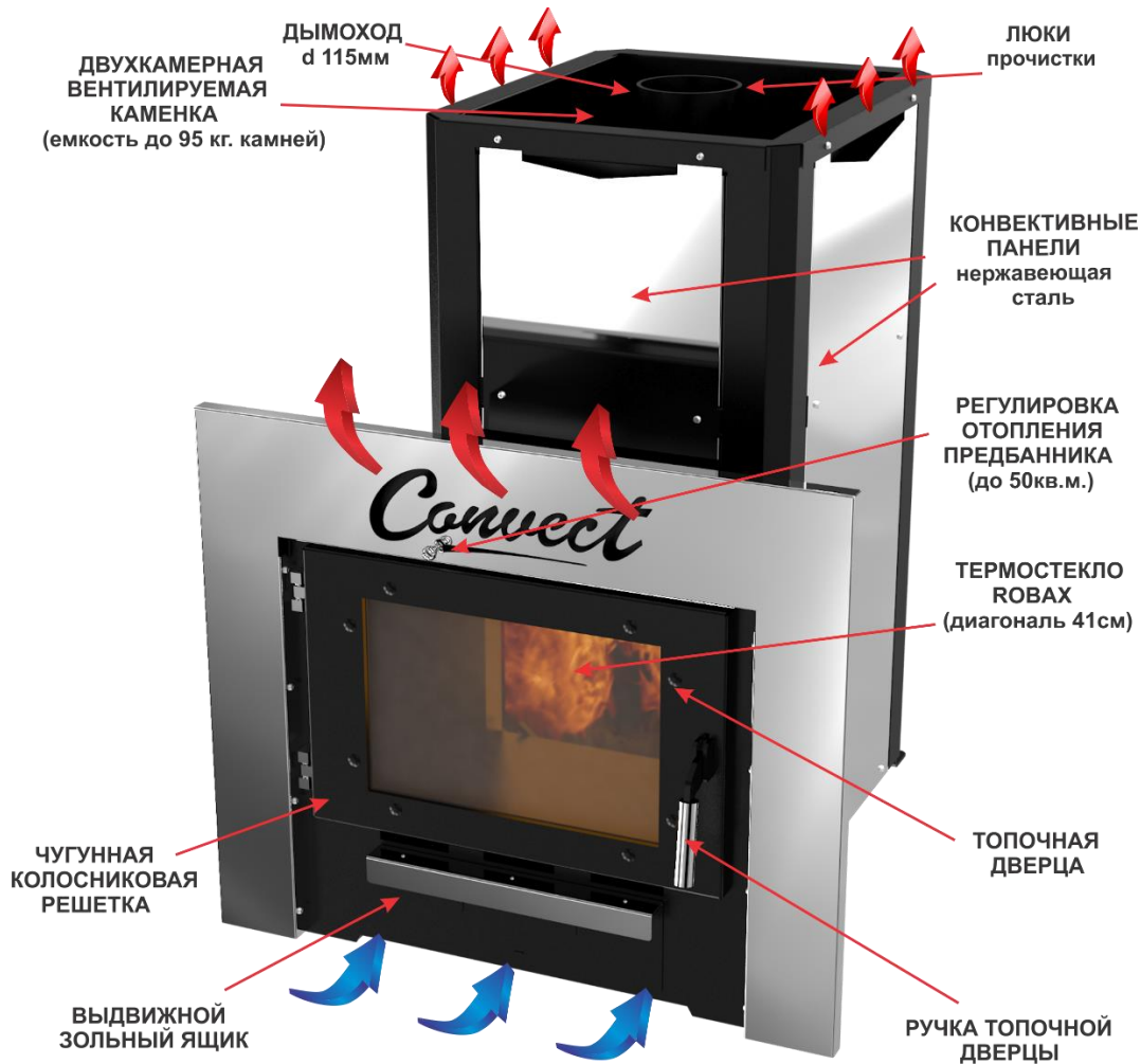
Рис. 2 Устройство печи CONVECT
