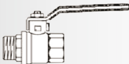
КРАН ШАРОВОЙ МУФТА/РЕЗЬБА ПОЛНОПРОХОДНОЙ (РЫЧАГ)
