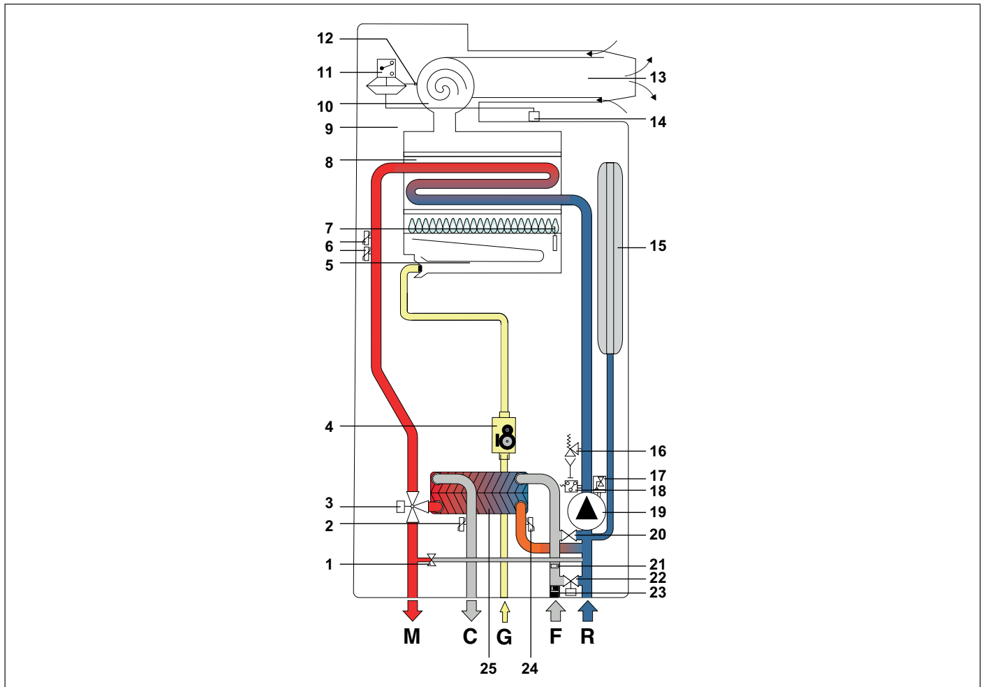
Рис. 8 Гидравлические схемы CTFS
