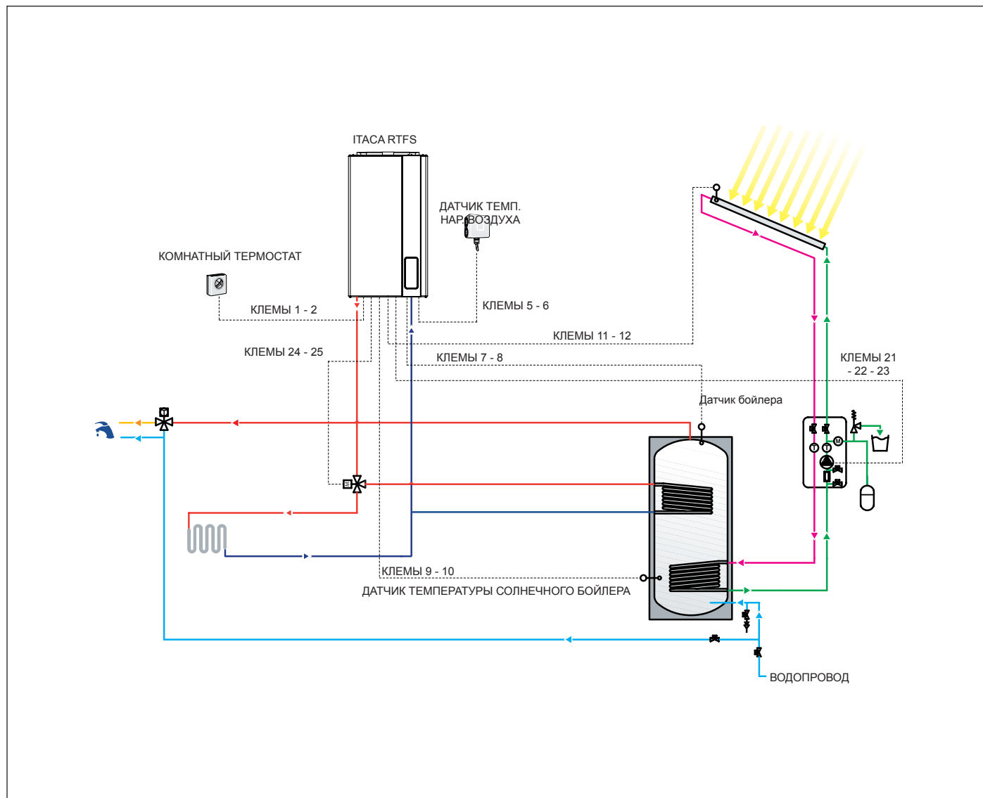
Рис. 22 Схема подключения системы солнечных коллекторов с принудительной циркуляцией к одноконтурному котлу
