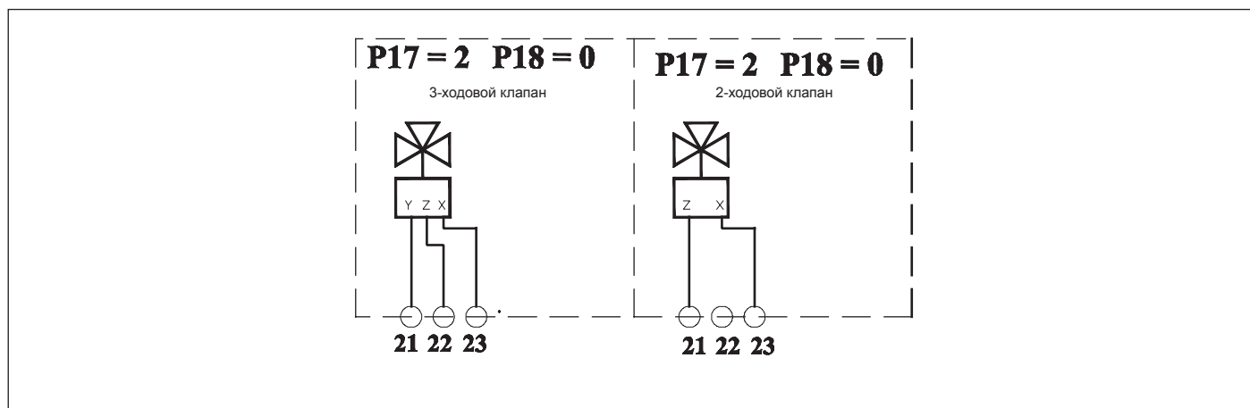
Рис. 29 Схема подключения многофункционального реле (X = общий; Y = на котел; Z = на коллектор)
