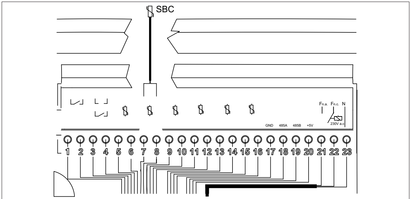
Рис. 21 Подробная электрическая схема RBTF5
