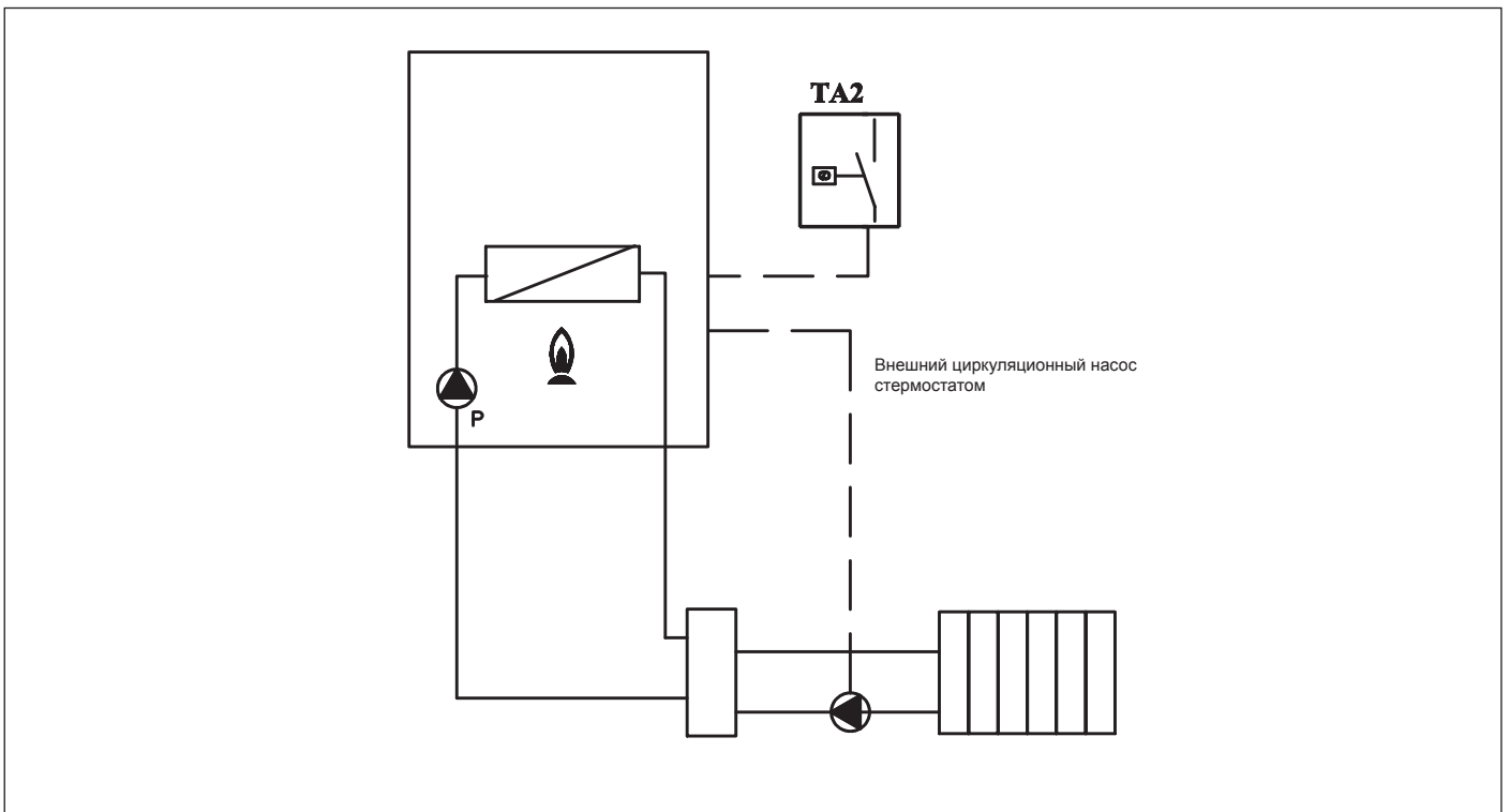
Рис. 33 Работа реле по внешнему запросу (P17=3)
