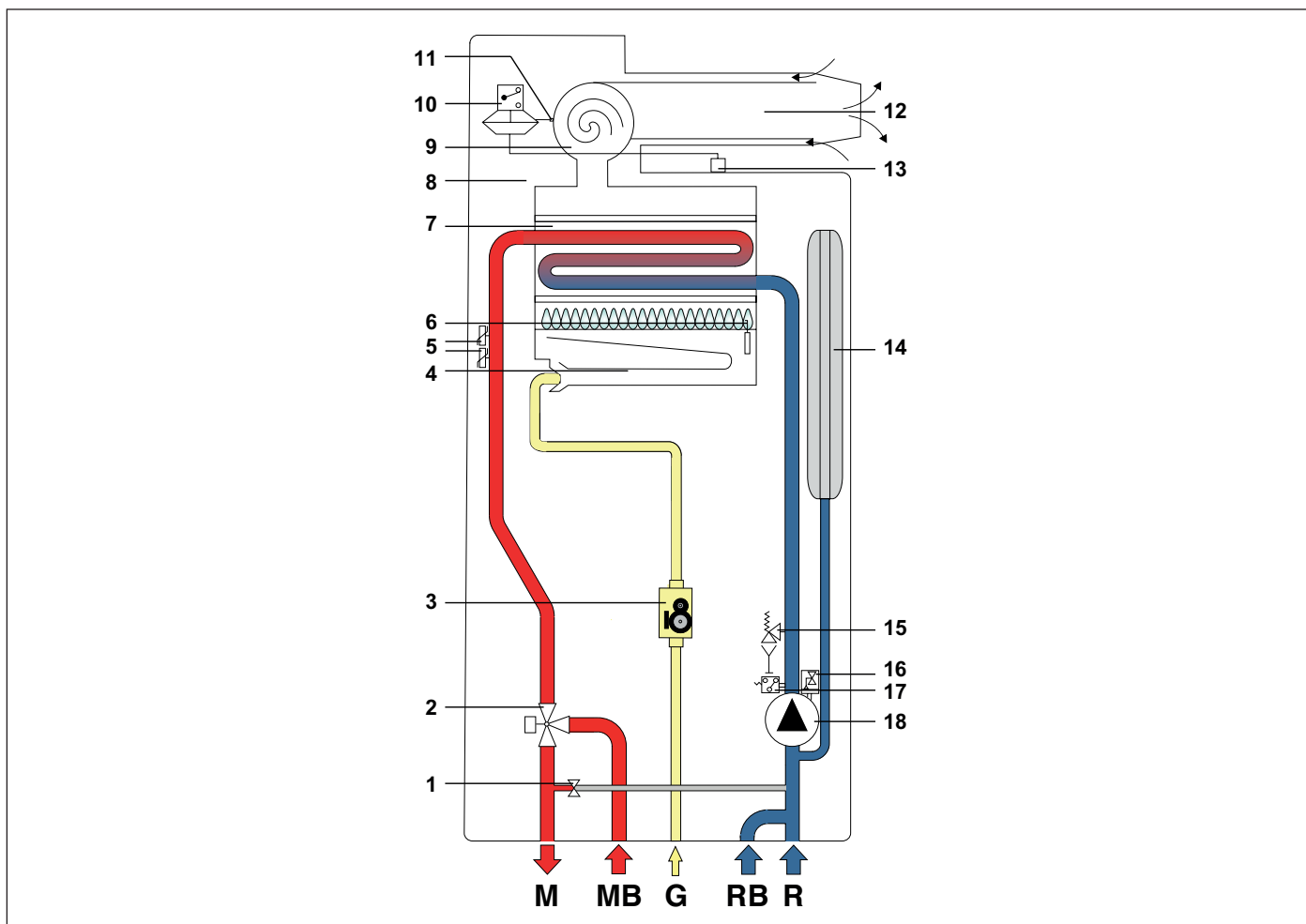
Рис. 7 Гидравлические схемы RBTFS
