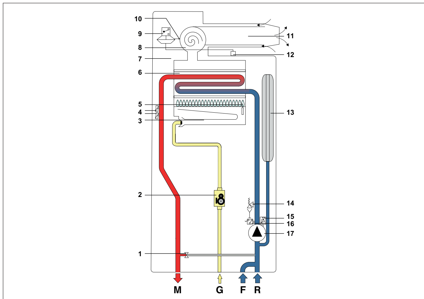
Рис. 6 Гидравлические схемы RTFS
