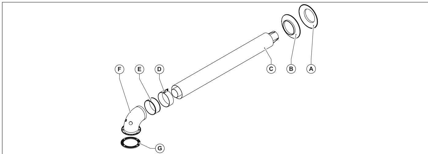
Рис. 10 Коаксильный комплект OKITCONC00
