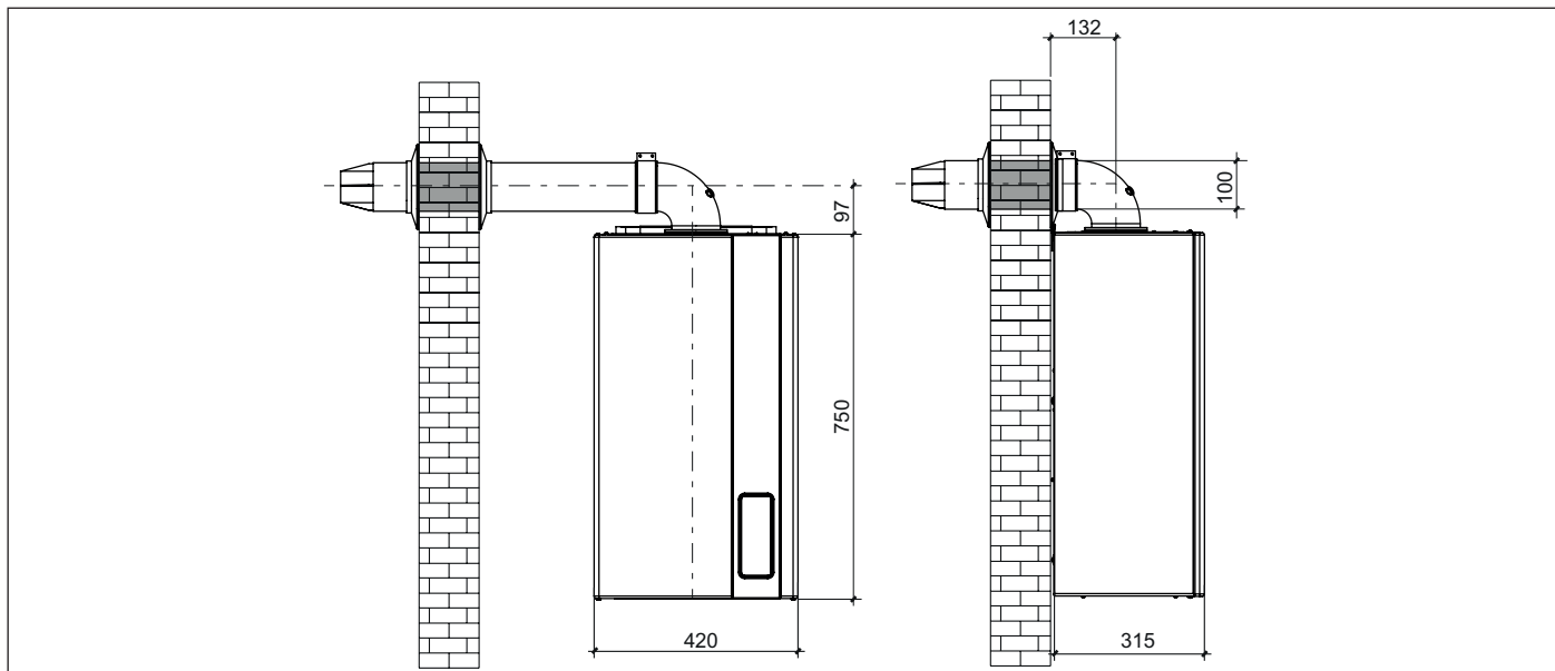
Рис. 12 Размеры для подсоединения к коаксиальному трубопроводу забора воздуха/отвода дымовых газов
