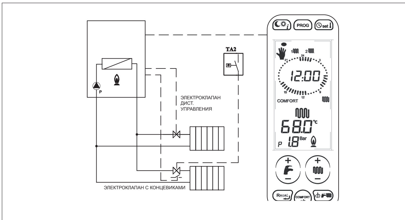
Рис. 31 Работа реле с панелью управления и TA2
