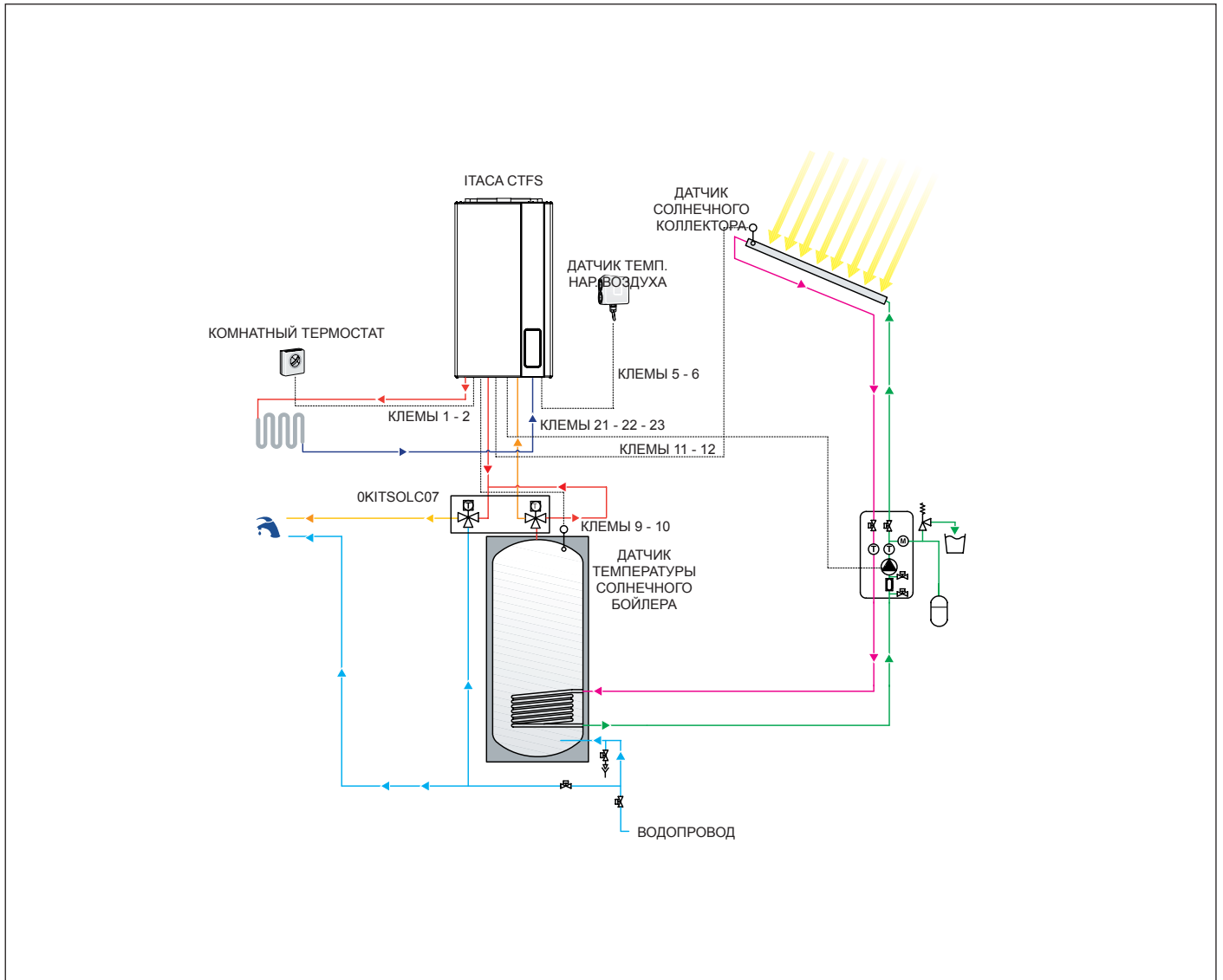
Рис. 26 Схема подключения системы солнечных коллекторов с принудительной циркуляцией к комбинированному котлу
