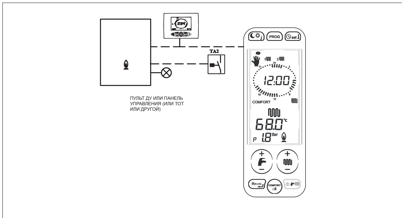
Рис. 34 Работа реле в схеме диспетчеризации (P17=0)
