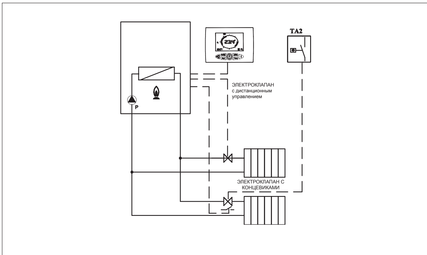
Рис. 30 Работа Реле с пультом ДУ и TA2
