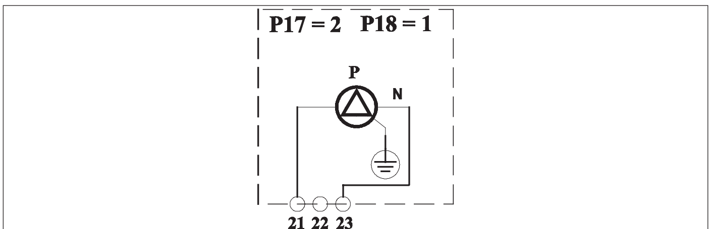
Рис. 27 Схема подключения многофункционального реле
