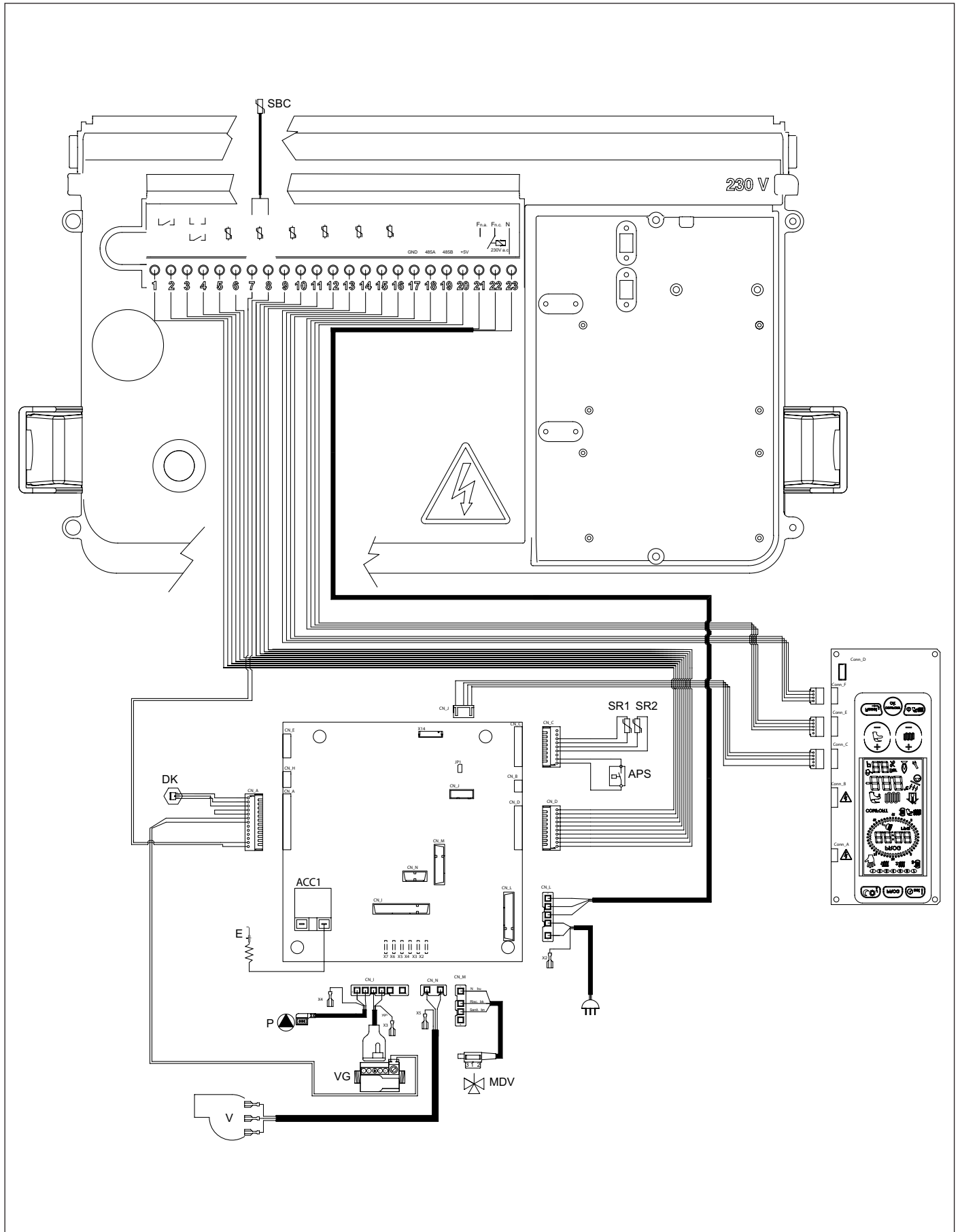
Рис. 20 Электрическая схема RBTFS
