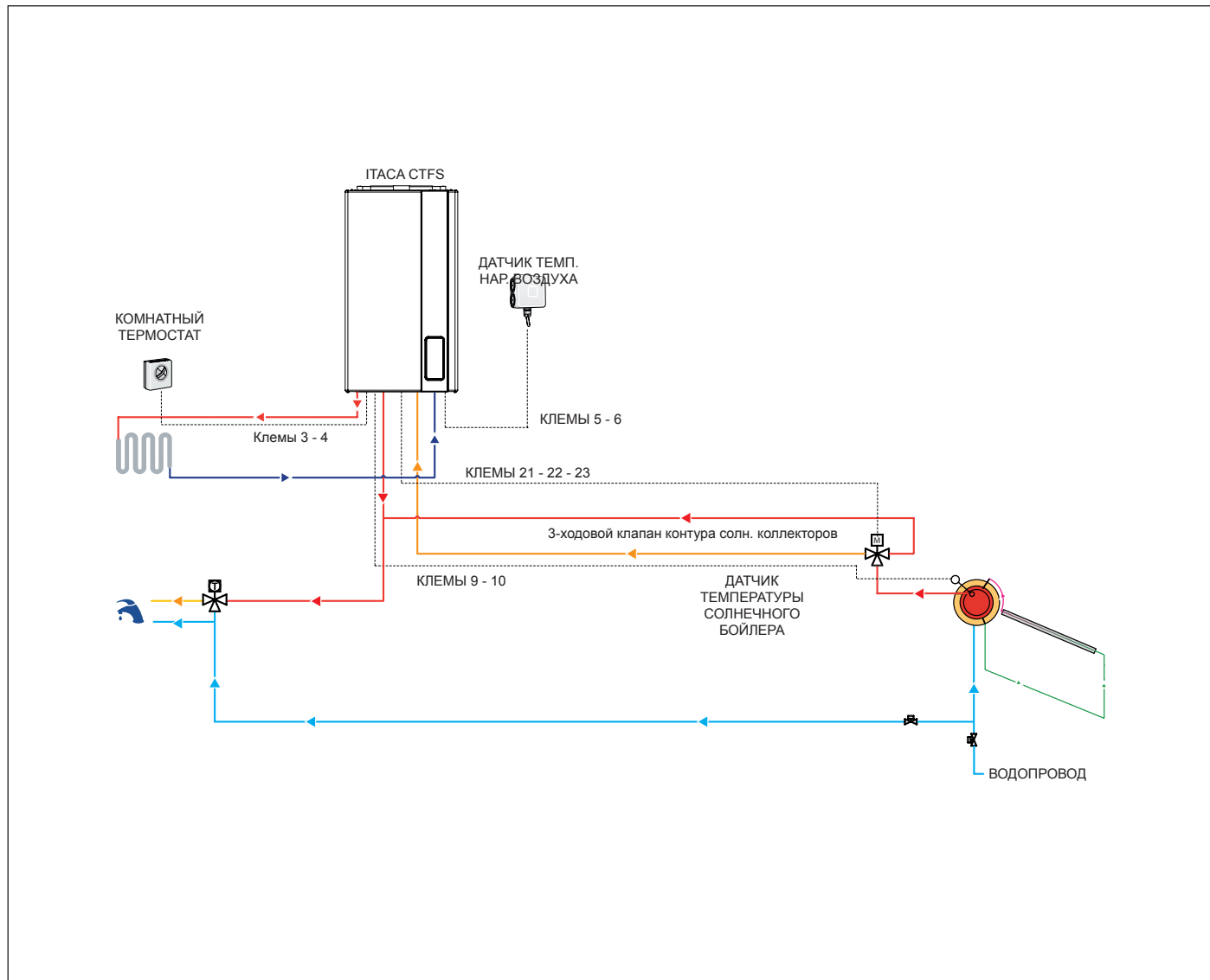
Рис. 28 Схема подключения системы солнечных коллекторов с естественной циркуляцией к комбинированному котлу
