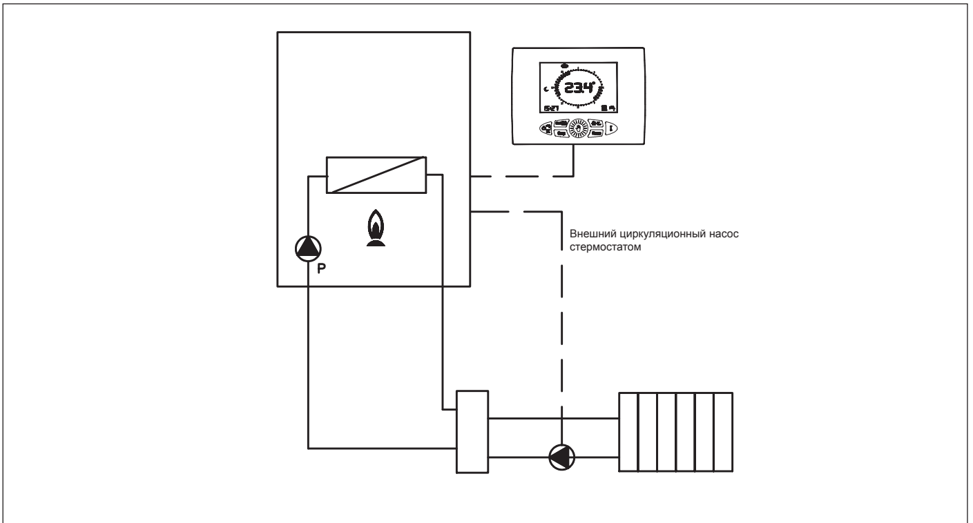
Рис. 32 Работа реле по внешнему запросу (P17=1)
