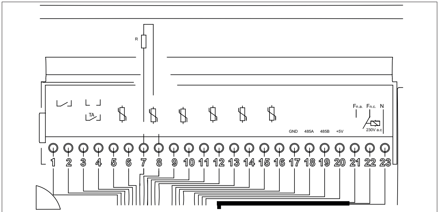
Рис. 19 Подробная электрическая схема RTFS
